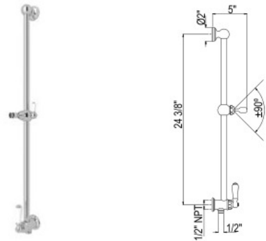
Rail de douche 26" 26" Slide Bar
