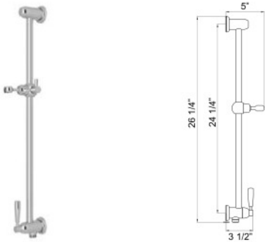
Rail de douche 25" avec contrôle de volume et sortie de douchette intégré Ed 25" Slide Bar With Integrated Volume Control And Outlet
