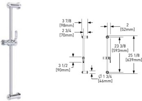
Rail de douche 26" 26" Slide Bar
